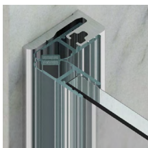
Dichtprofil Glas-Wand mit Trägerprofil sealing profile glass wall with support profile
