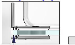
Duschtürband 8406MS einseitige Befestigungslasche
