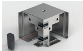
Eckverbinder Seitenteil/Türflügel corner connector side panel/door Art.-Nr.: | art. no.: 8822ZN_EST90
