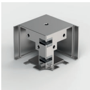
Eckverbinder für Seitenteil/Seitenteil corner connector for side panel/side panel Art.-Nr.: | art no.: 8822ZN_-ESS90
