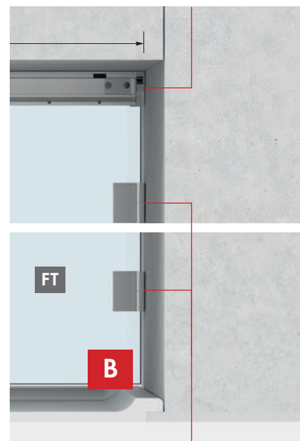
Wandhalter am Seitenteil wall bracket on the side panel Art.-Nr.: | art. no.: 8822ZN_EL/ER
