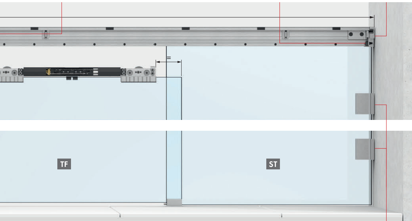
Wandhalter am Seitenteil wall bracket on the side panel Art.-Nr.: | art no.: 8822ZN_-EL/ER
