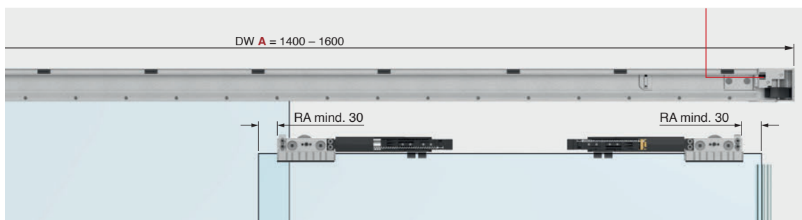
2x Softstopp einseitig (32 kg) 2x softstopp single-sided (32 kg) Art.-Nr.: | art. no.: 8822RAL7016-SSD-32
