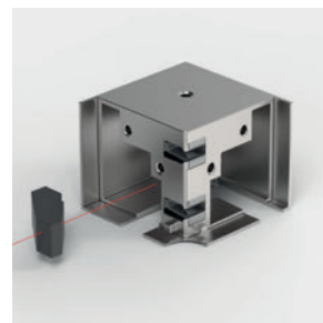
Eckverbinder für Seitenteil/Tür corner connector for side panel/door Art.-Nr.: | art no.: 8822ZN_-EST90L/R
