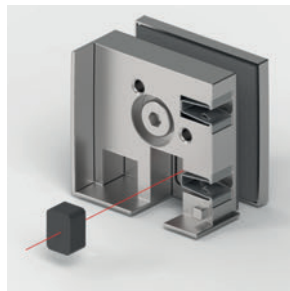
Glashalterung am Durchgang glass bracket at the doorway Art.-Nr.: | art no.: 8822ZN_-GL/GR
