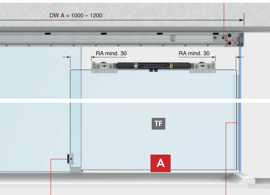
Eckverbinder Seitenteil/Türflügel corner connector side panel/door Art.-Nr.: | art. no.: 8822ZN_EST90
