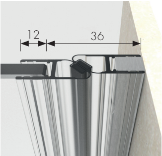
N° d'Art. | Art.-no. 8852KU0-8-2010 Transparent
