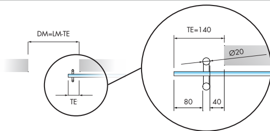
Un vantail + partie fixe
