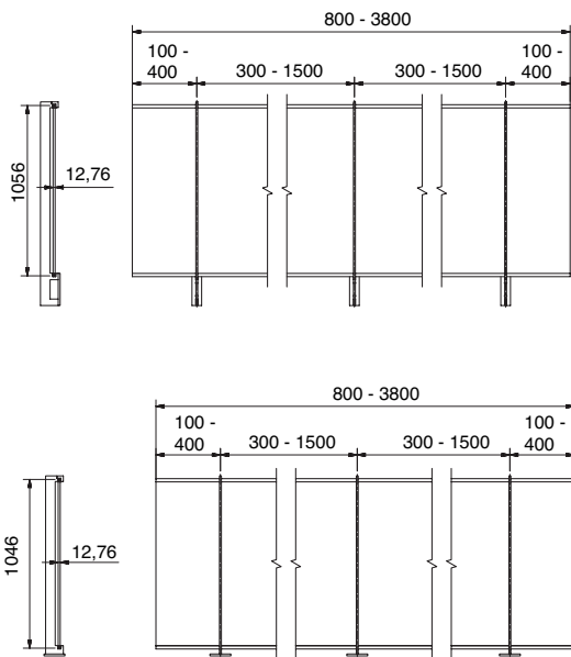
Dimensions système de balustrade avec 3 piliers
