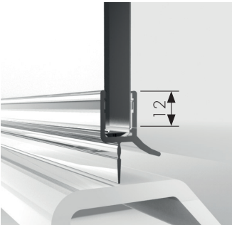
N° d'Art. | Art.-no. 8864KU0-8-2010 Transparent
