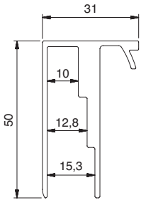
Raccord panneaux de cloison sèche pour 1402
