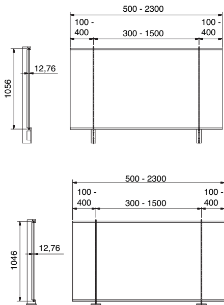
Dimensions système de balustrade avec 2 piliers
