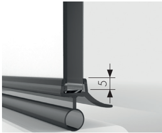
N° d'Art. | Art.-no. 8863KU0-8K-2010 Transparent 8863KU3-8K-2010 Noir
