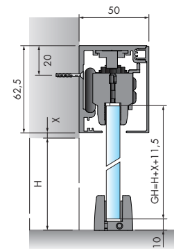
Set de portes coulissantes sans partie latérale, fixation murale
