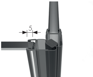
N° d'Art. | Art.-no. 8851KU0-8K-2500 Transparent 8851KU3-8K-2500 Noir
