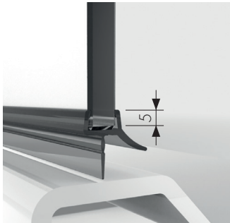
N° d'Art. | Art.-no. 8864KU0-8K-2010 Transparent 8864KU3-8K-2010 Noir
