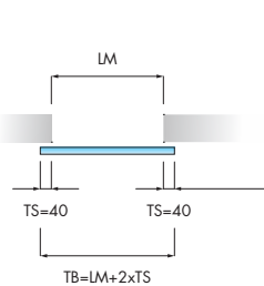
À un vantail
