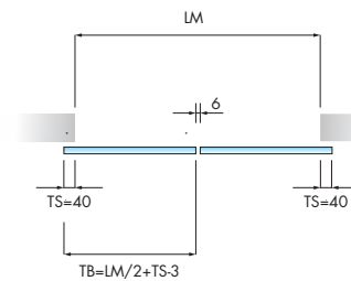
À deux vantaux
