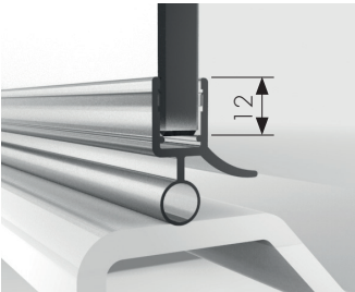
N° d'Art. | Art.-no. 8863KU0-8-2010 Transparent
