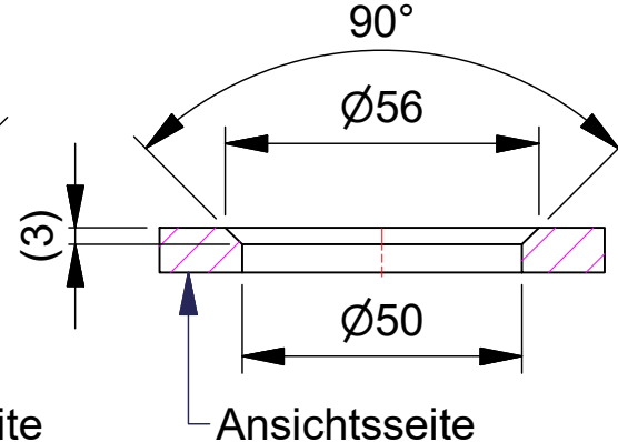
D-D
