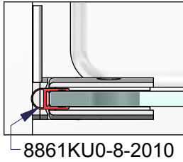
Duschtürband 8406MS einseitige Befestigungslasche
