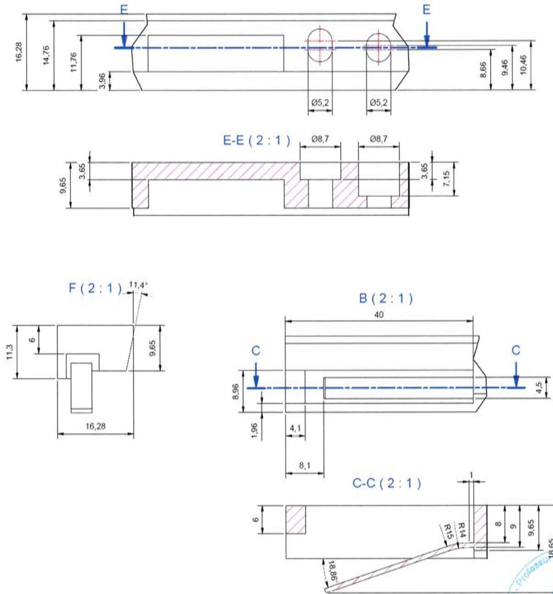
Abbildung 52 Artikelnummer 1440-152KU: Kunststoffdruckleiste für VSG mit 1,52 mm Zwischenschicht
