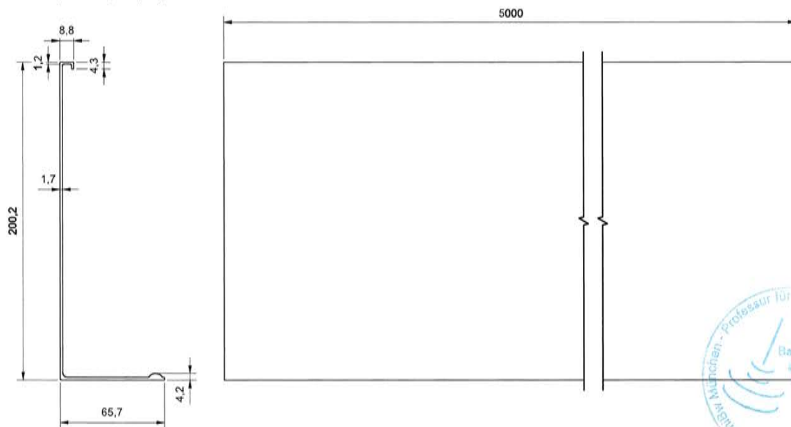
Abbildung 31 Artikelnummer 1442-2R-5: Blende für Systemprofil
