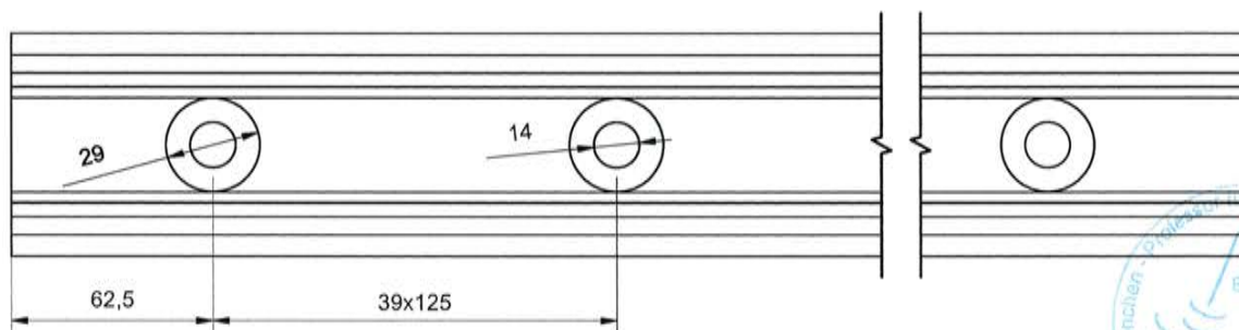
Abbildung 50 Artikelnummer 1444-1R-17/21-5 Grundprofil für Bodenmontage aufgesetzt, für VSG 16,76 / 17,52 (17) und VSG 20,76 / 21,52 (21)
