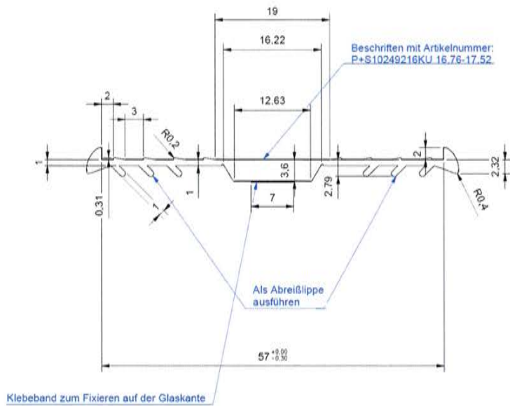
Abbildung 58 Artikelnummer 10249216KU: Verglasungsprofil für U-Profil 26x24x2
