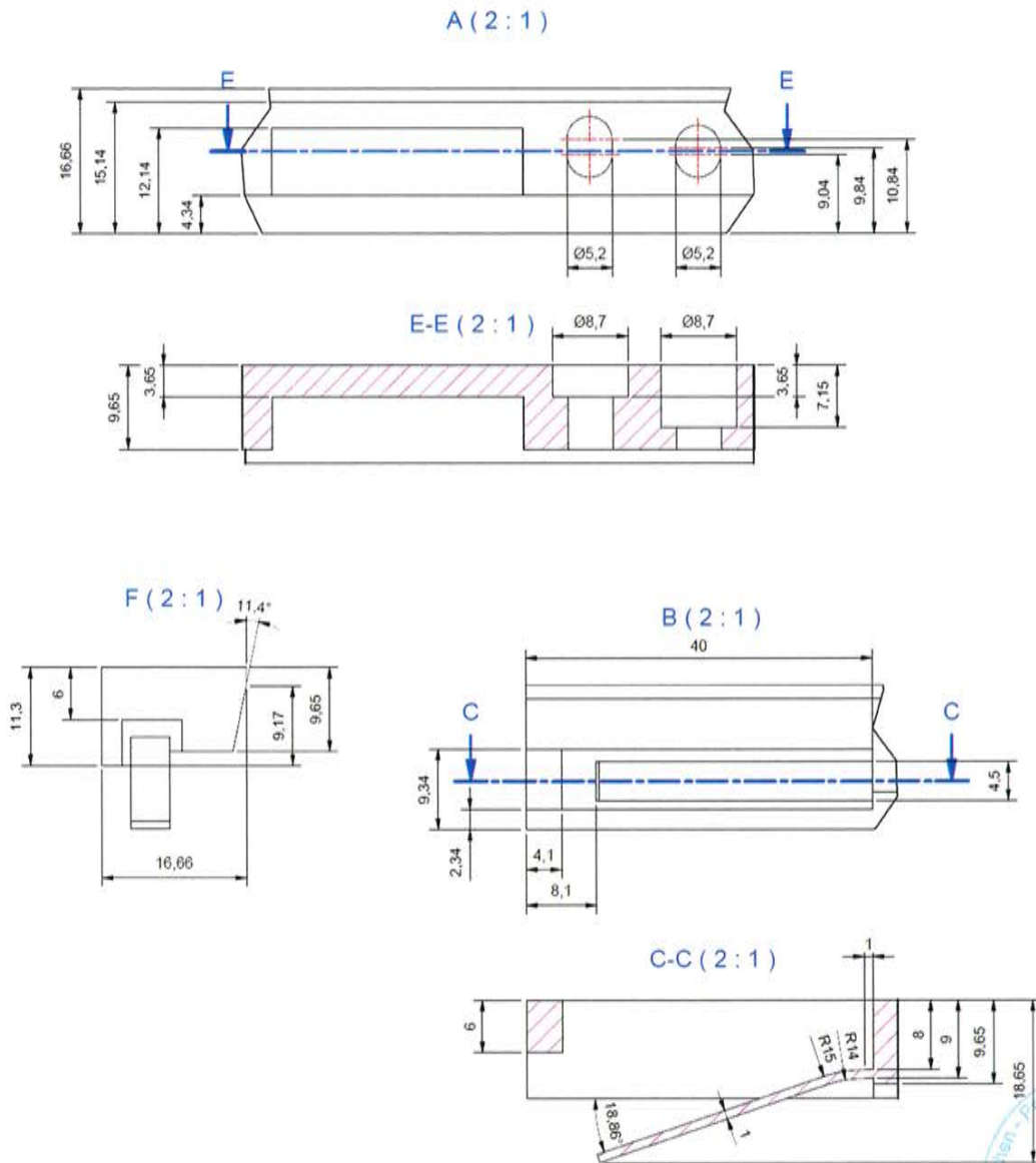
Abbildung 51 Artikelnummer 1440-076KU: Kunststoffdruckleiste für VSG mit 0,76 mm Zwischenschicht
