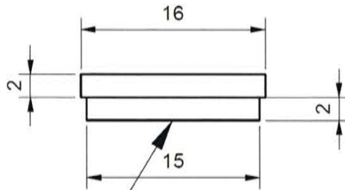
Abbildung 65 Artikelnummer 7268E0-12: Kantenschutzprofil VSG 12
