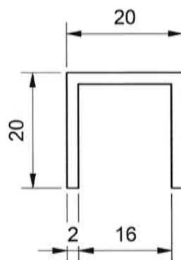
Abbildung 63 Artikelnummer 5020E0: Kantenschutzprofil U-Profil 20x20x2 mm für Glas 10-12 mm
