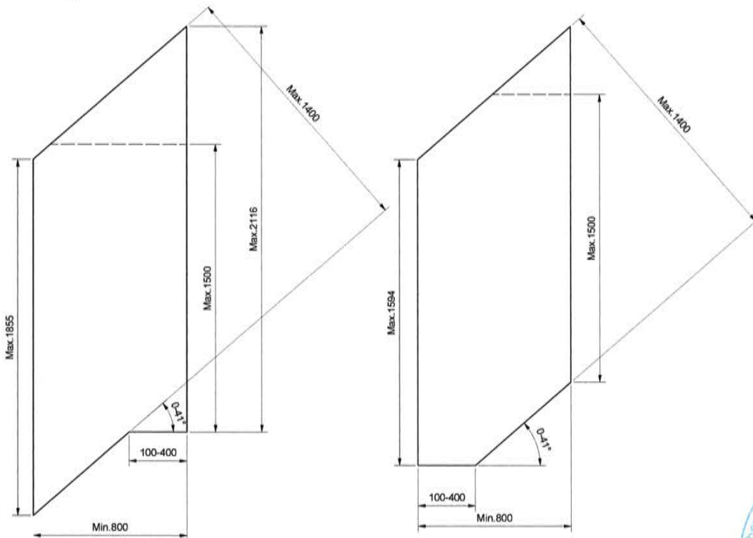
Abbildung 8 Aufbau 10 mm ESG / 0,76 mm PVB bzw. 1,52 mm PVB / 10 mm ESG, Angaben zu Bohrungen siehe Tabelle 3 bis Tabelle 5
