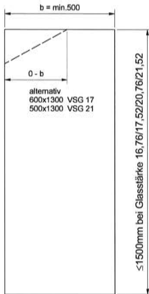
Abbildung 6 Aufbau Rechteckscheiben 8 mm ESG / 0,76 mm PVB bzw. 1,52 mm PVB / 8 mm ESG und 10 mm ESG / 0,76 mm PVB bzw. 1,52 mm PVB / 10 mm ESG, Angaben zu Bohrungen siehe Tabelle 2
