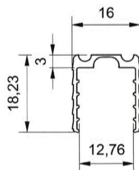
Abbildung 64 Artikelnummer 10245320KU: Gummiprofil für U-Profil 5020 für Glas 12 mm
