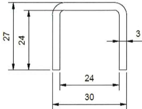
Abbildung 55 Artikelnummer 5022VA4: U-Profil 27 x 30 x 3 mm
