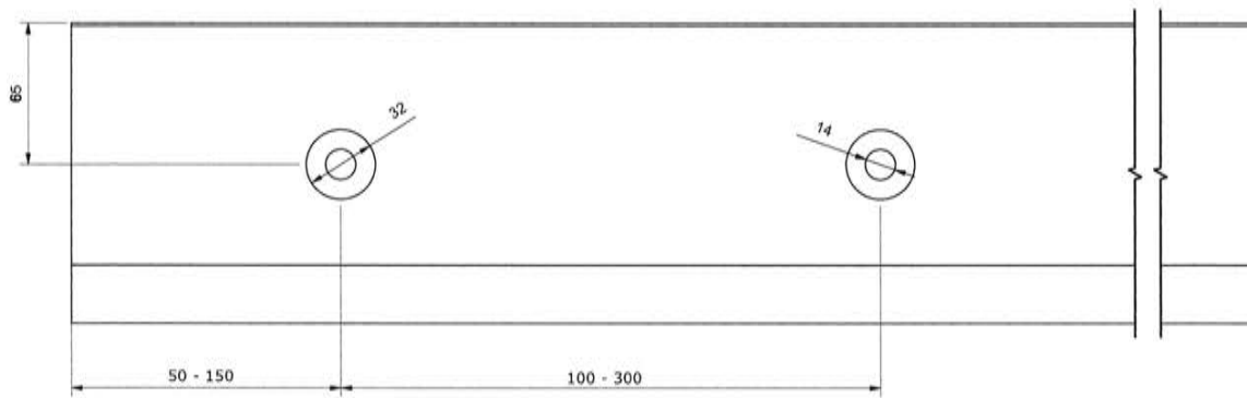
Abbildung 40 Artikelnummer 1443-1R-17/21-5 Grundprofil für Frontmontage, für VSG 16,76 / 17,52 (17) und VSG 20,76 / 21,52 (21)
