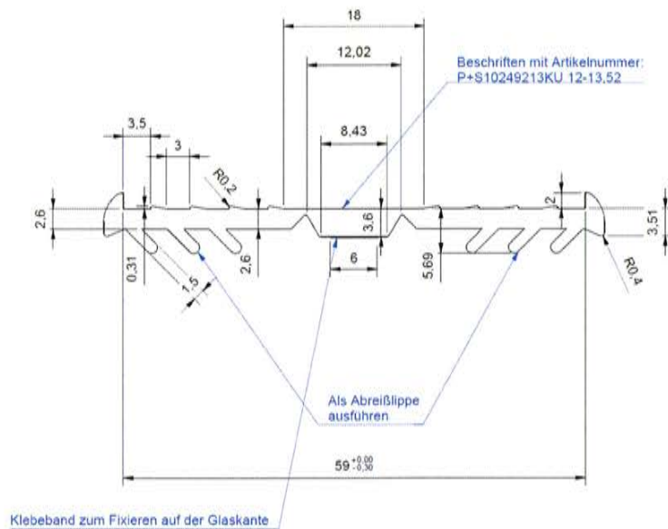
Abbildung 57 Artikelnummer 10249213KU: Verglasungsprofil für U-Profil 26x24x2, Glasdicke 12-13,52 mm
