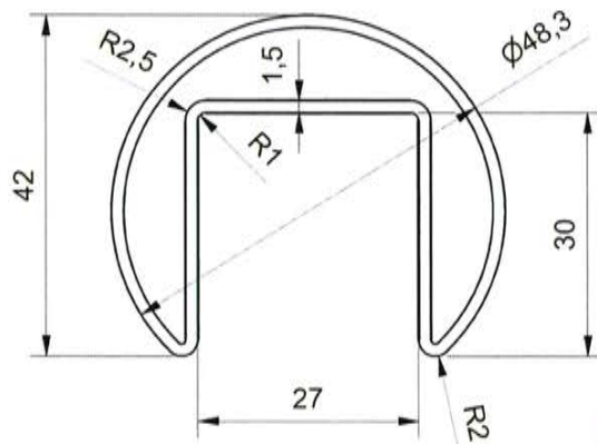
Abbildung 54 Artikelnummer 10242648A4: Handlauf Nutrohr \varnothing 48,3 mm
