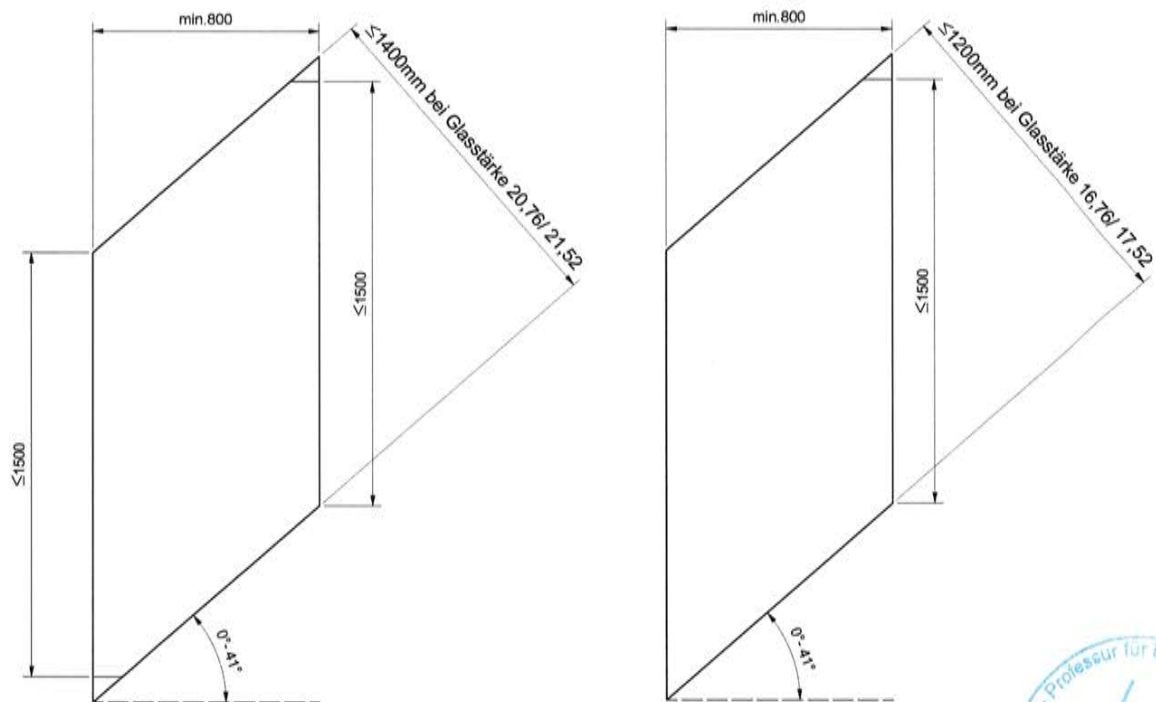
Abbildung 7 Aufbau Parallelogrammscheiben 10 mm ESG / 0,76 mm PVB bzw. 1,52 mm PVB / 10 mm ESG (links) und 8 mm ESG / 0,76 mm PVB bzw. 1,52 mm PVB / 8 mm ESG (rechts), Angaben zu Bohrungen siehe Tabelle 3 bis Tabelle 5
