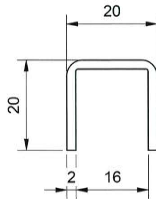
Abbildung 62 Artikelnummer 5020VA: Kantenschutzprofil U-Profil 20x20x2 mm für Glas 10-12 mm
