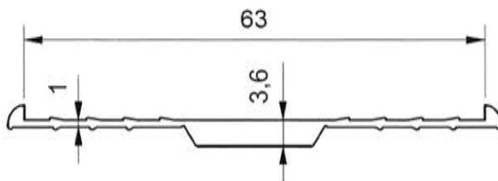
Abbildung 59 Artikelnummer 10214842KU: Elastomer-Profil für Nutsysteme für Glas 20,76-21,52 mm
