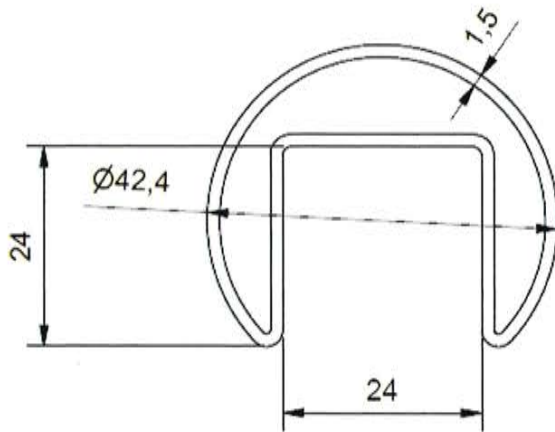
Abbildung 53 Artikelnummer 10242642A2/A4: Handlauf Nutrohr \varnothing 42,4 mm
