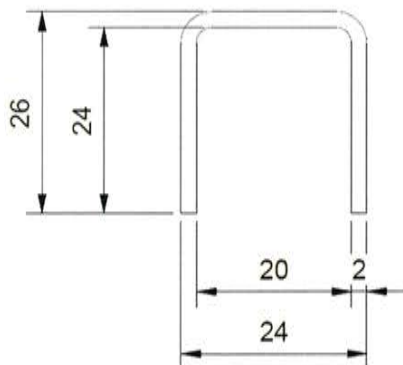
Abbildung 56 Artikelnummer 5021VA4: U-Profil 26 x 24 x 2 mm
