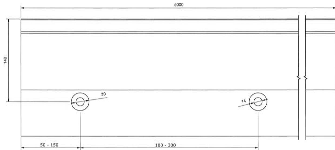
Abbildung 30 Artikelnummer 1442-1R-17/21-5 Grundprofil für Frontmontage, für VSG 16,76 / 17,52 (17) und VSG 20,76 / 21,52 (21)
