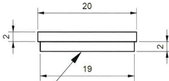
Abbildung 66 Artikelnummer 7268E0-16: Kantenschutzprofil VSG 16
