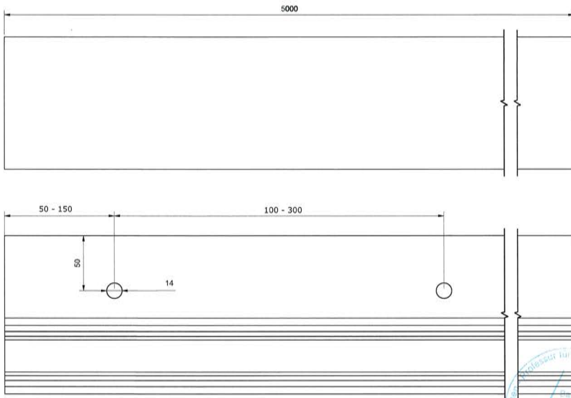
Abbildung 19 Artikelnummer 1440-1R-17/21-5 Verglasungsprofil, Bodenmontage aufgesetzt mit seitlicher La- sche, für VSG 16,76 / 17,52 (17) und VSG 20,76 / 21,52 (21)
