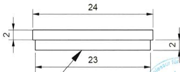
Abbildung 67 Artikelnummer 7268E0-20: Kantenschutzprofil VSG 20
