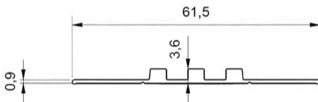
Abbildung 60 Artikelnummer 10245448KU: Elastomer-Profil für Nutsysteme für Glas 25,52 mm
