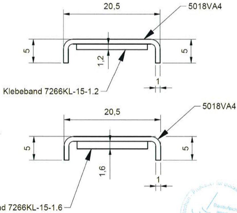
Abbildung 61 Artikelnummer 5018VA4: Kantenschutzprofil U-Profil 5x20,5x1 mm
