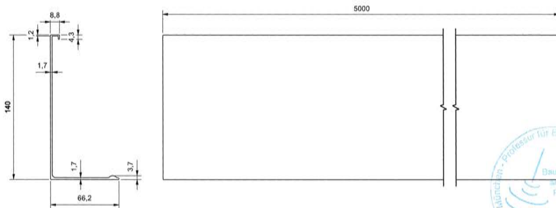
Abbildung 41 Artikelnummer 1443-2R-5: Blende für Systemprofil
