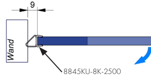
Glasbearbeitung 8354ZN mit Dichtung 8845KU0-8K
