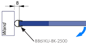
Glasbearbeitung 8350ZN mit Dichtung 8861KU0-8K
